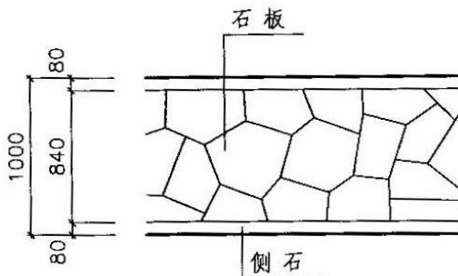
冰纹路游步道铺装平面图
