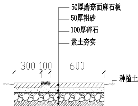
石板嵌草路剖面图
