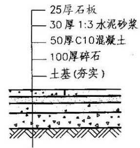
冰纹路游步道铺装剖面图
