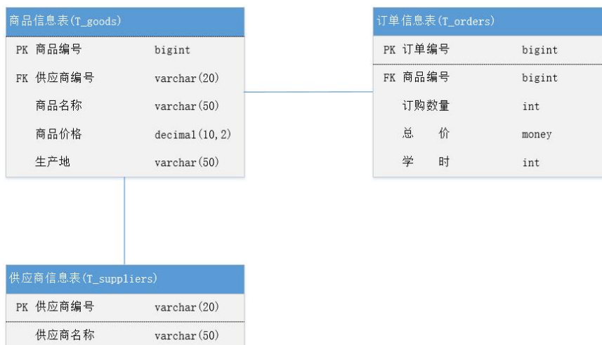
图 2.6.2 物理数据模型图
