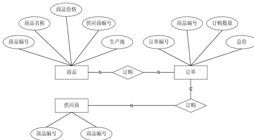
图 2.5.1 E-R 图
