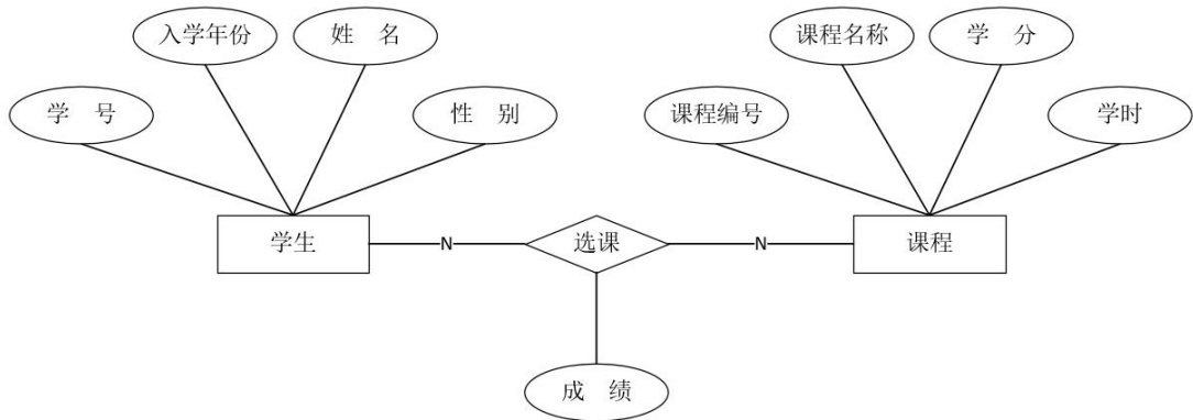
图 2.3.1 E-R 图
