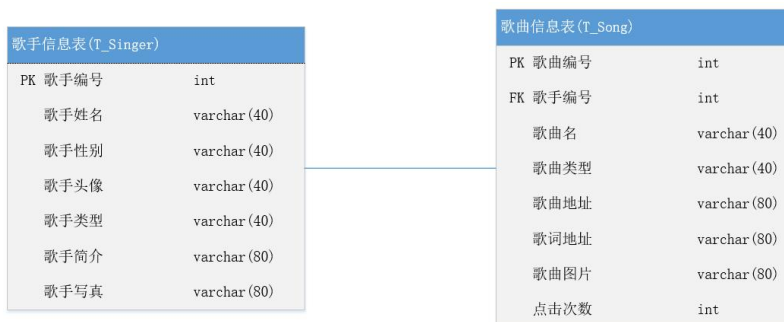
图 2.13.2 物理数据模型图
