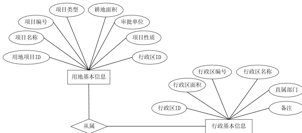
图 2.7.1 E-R 图
