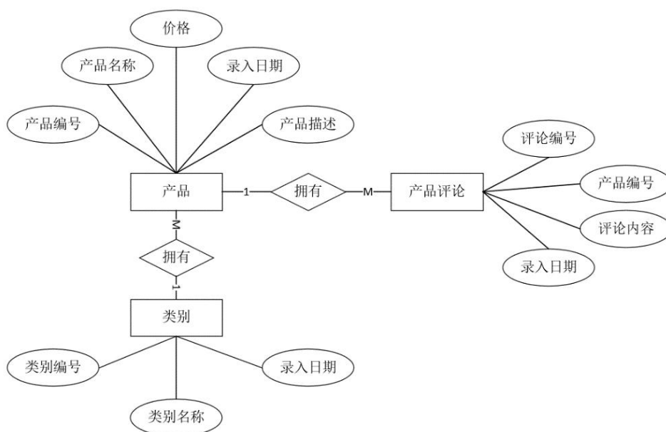
图 2.2.1 E-R图
