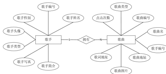
图 2.13.1 E-R 图
