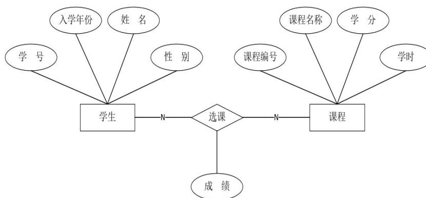
图 2.4.1 E-R 图
