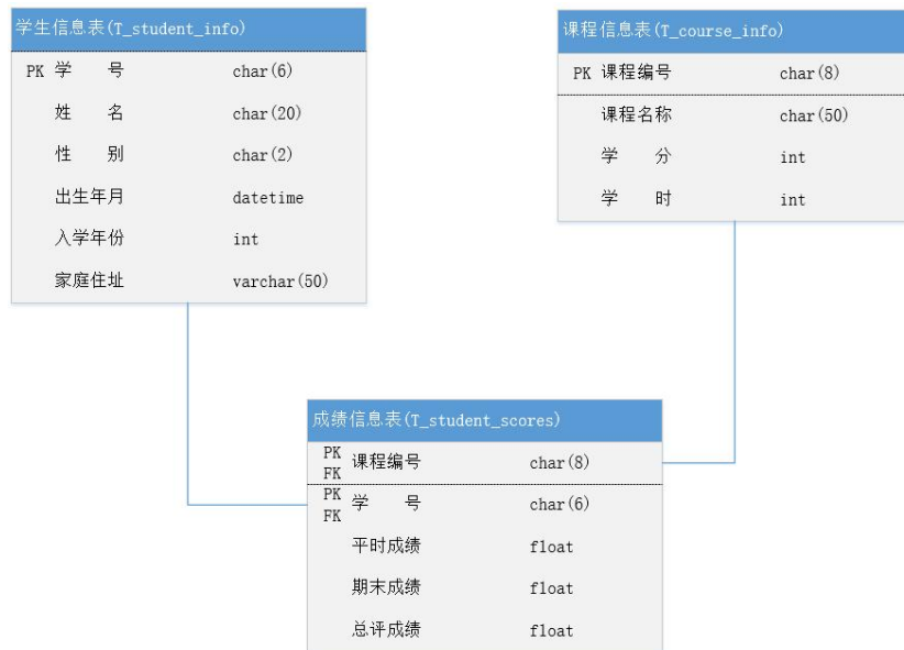
图 2.3.2 物理数据模型图
